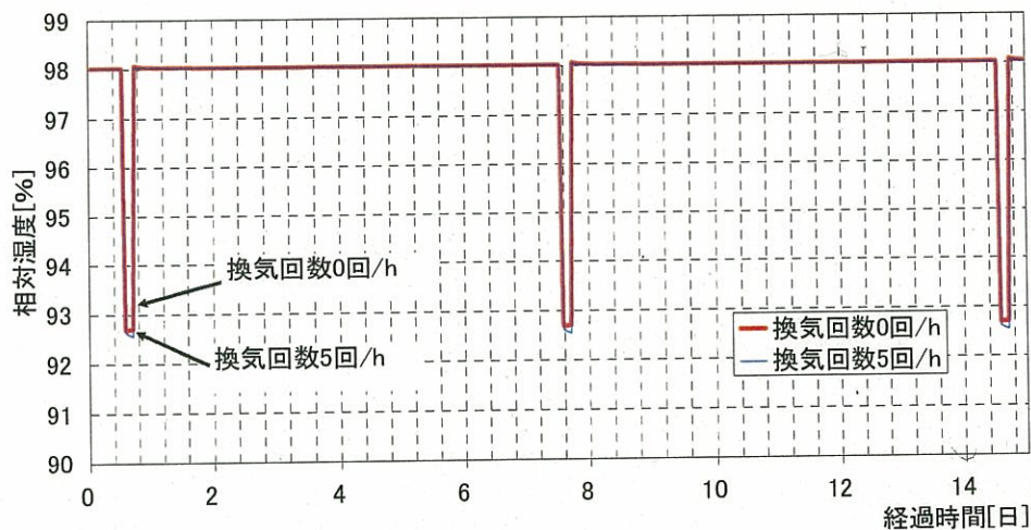
図 4 石室内相対湿度変動（発熱量 60W）
