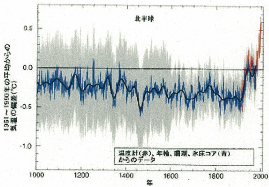
図 6 - 3 北半球における過去 1000 年間の年平均気温の経年変化（地球温暖化） （IPPC 第三次報告書より）
